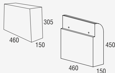
ОПОРА «ГАРДЕН 3» Арт: 607091011.046030 (промежуточная), масса 50 кг Арт: 607091011.046045 (крайняя), масса 70 кг Единица измерения: штука
