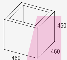
ВАЗОН «CUBE 44»
