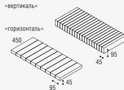
СИДЕНЬЕ «ВЕРТИКАЛЬ»/«ГОРИЗОНТАЛЬ» (дерево) Арт.: 608355972 («вертикаль»), масса 13 кг Арт.: 608345972 («горизонталь»), масса 7 кг Единица измерения: метр
