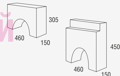
ОПОРА «SP-GAMMA3» Арт: 607071011.046030 (промежуточная), масса 40 кг Арт: 607071011.046045 (крайняя), масса 60 кг Единица измерения: штука
