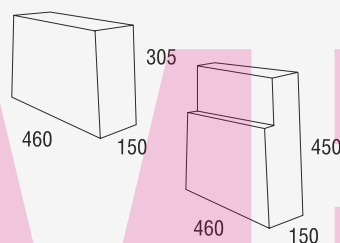
ОПОРА «SP-ALFA» Арт: 607031011.046030 (промежуточная), масса 50 кг Арт: 607031011.046045 (крайняя), масса 72 кг Единица измерения: штука
