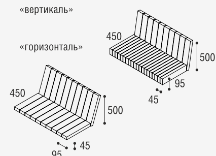
СИДЕНЬЕ СО СПИНКОЙ (дерево) Арт.: 609355972 («вертикаль»), масса 19 кг Арт.: 609345972 («горизонталь»), масса 14 кг Единица измерения: метр
