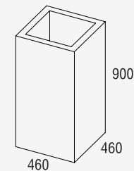
ВАЗОН «CUBE 49»
