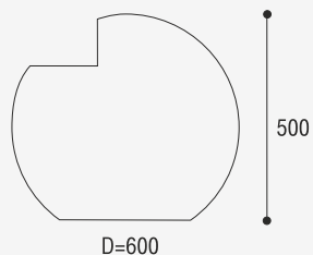
ОПОРА «BALL» Арт.: 607011011.060050 (бетон с закладными) Масса 250 кг Единица измерения: штука
